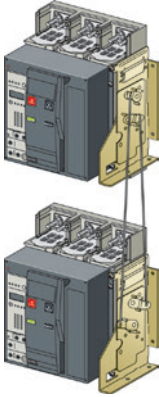
Çubuk ile dikey mekanik kilitleme
